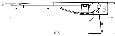
Вертикальное размещение
