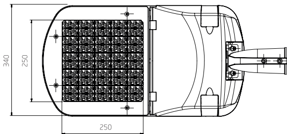
Горизонтальное размещение
